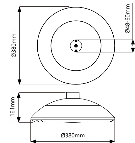
Dimensioni : NEWTON20 S SMALL - Attacco a sospensione
